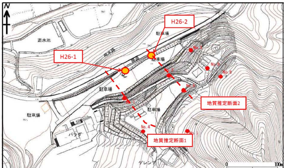
図 4-1-1 調査位置平面図
