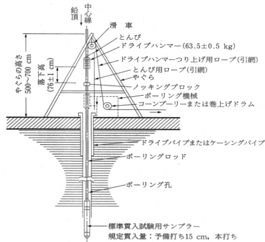
図 2-2-1 標準貫入試験装置および器具の名称 「地盤調査の方法と解説 (P251)：地盤工学会」より抜粋
