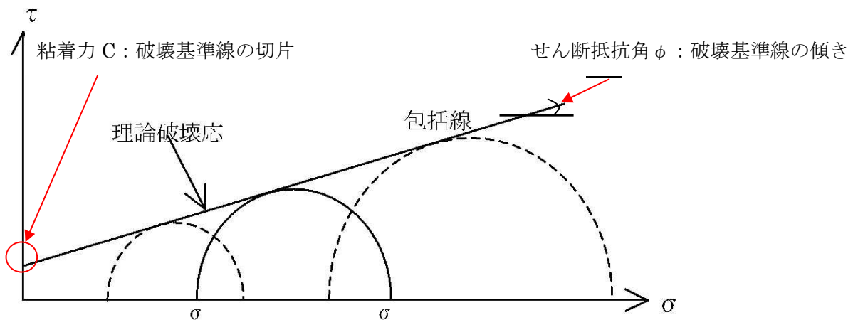
図 2-3-4 モール・クーロンの破壊基準
