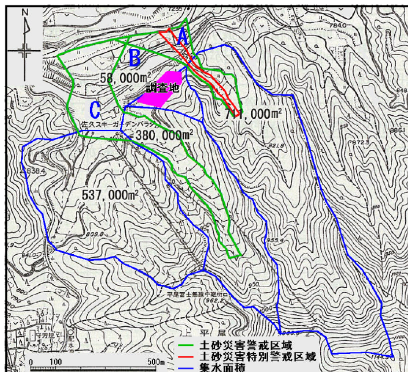
図 6-3-2 土砂災害警戒区域等と調査地との位置関係
