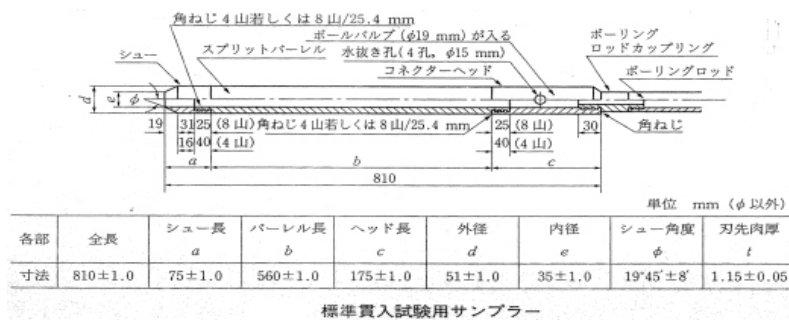
図 2-2-2 標準貫入試験用サンプラー 「地盤調査の方法と解説 (P247)：地盤工学会」より抜粋
