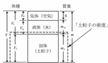
図 2-3-1 土の三相分布
