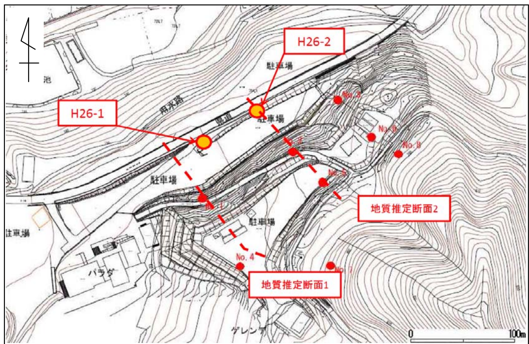
調査地平面図
