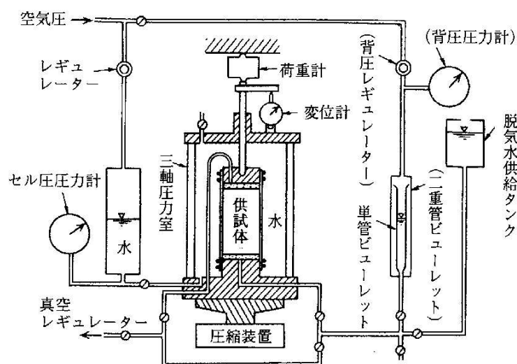
図 2-3-5 三軸圧縮試験機の構成例
