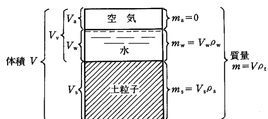
図 2-3-2 土を構成する 3 要素
