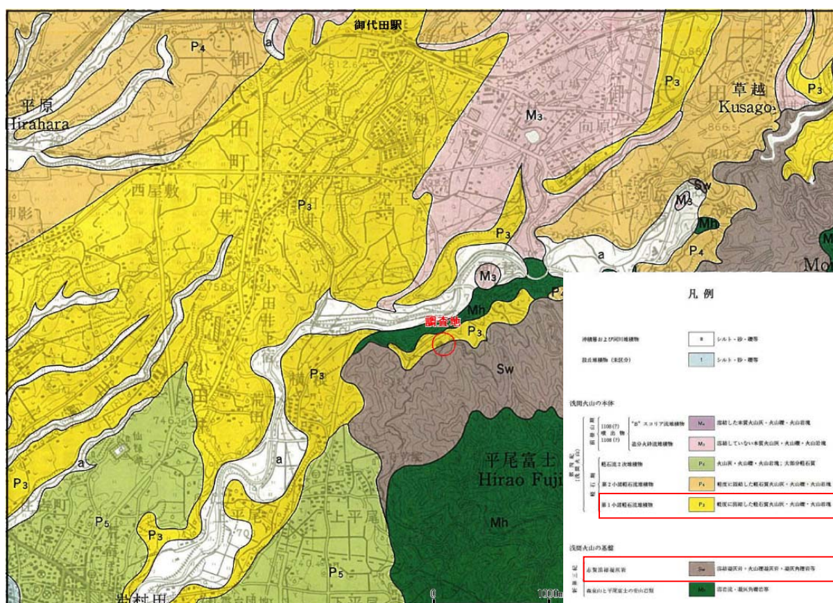
図 3-3 調査地周辺の地質図
